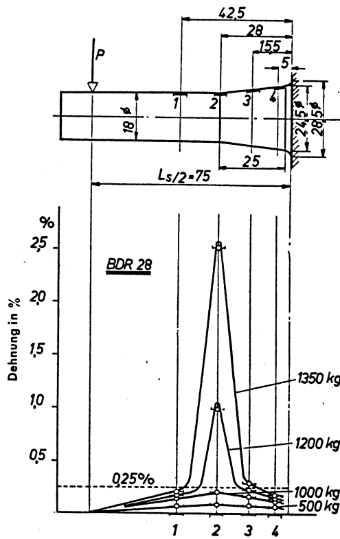
Abb. 2. Örtliche Dehnung des BDR 28 bei zunehmender Belastung
